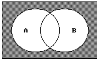
\overline{A} \cap \overline{B}
